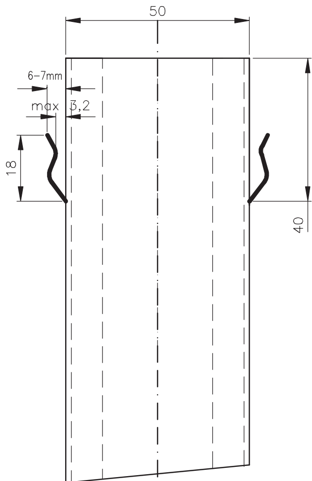
ŘEZ PROFILEM SLOUPKU
